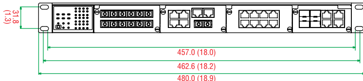
前视图
