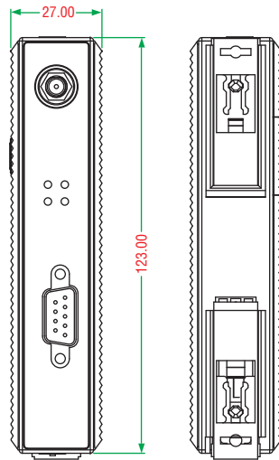
前视图&后视图
